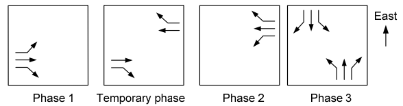
Fig. 7 Actual phase configuration
